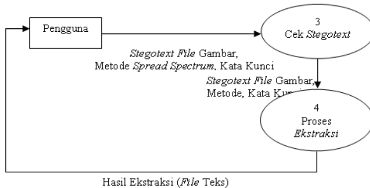
Gambar 3 DFD Level Satu Proses Ekstraksi Metode Spread Spectrum
